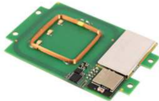
TWN4 MultiTech 2 BLE PCB top view
